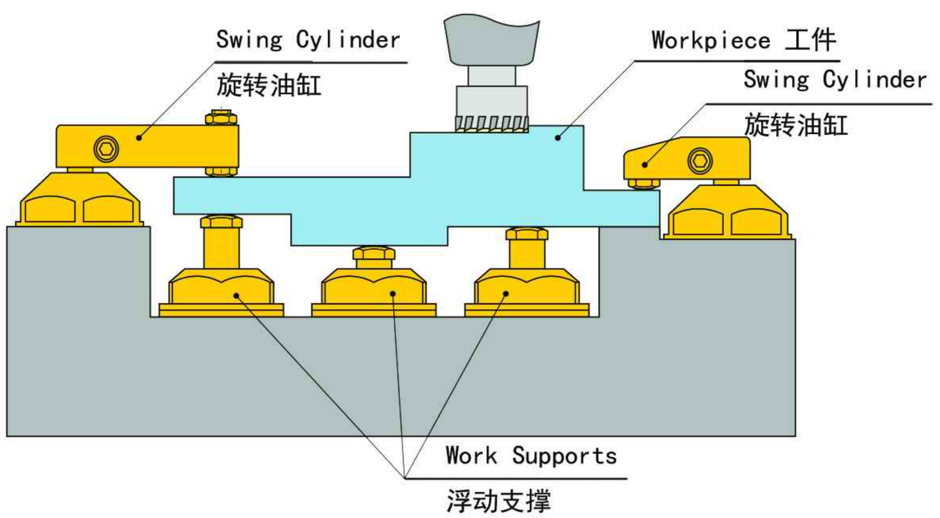
板式安装示意图
