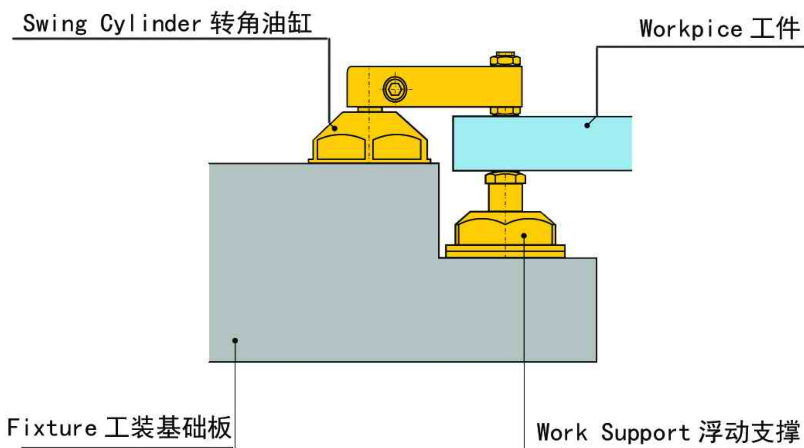
板式安装示意图
