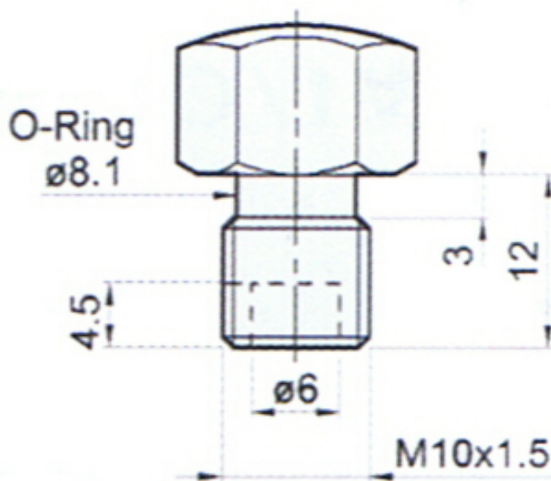
SP-16顶杆螺帽尺寸图
