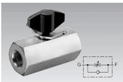
节流阀
