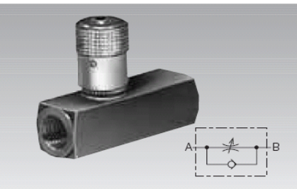
节流阀
