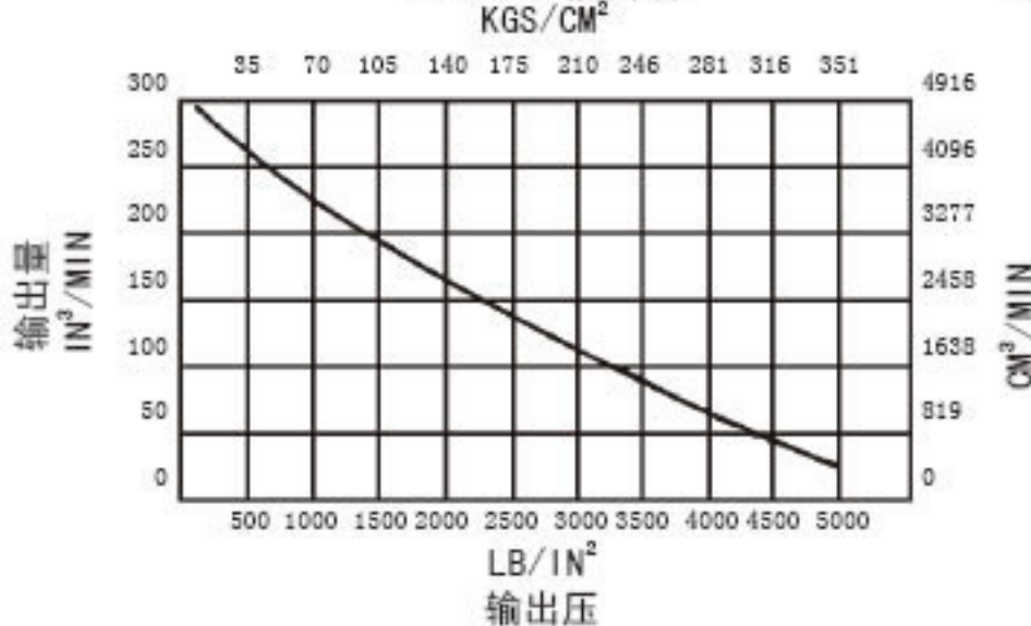
61762 性能曲线
