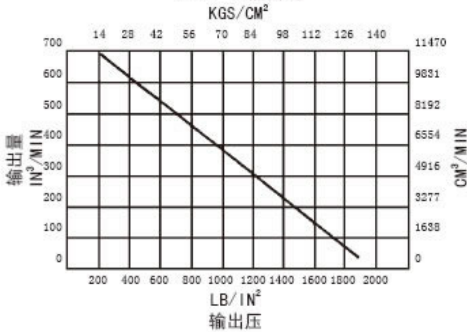
61761 性能曲线
